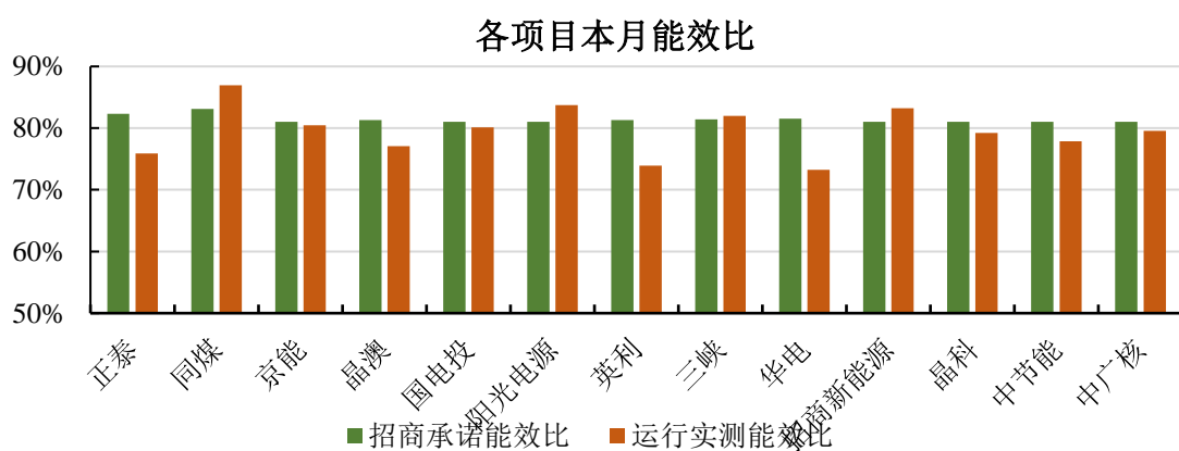
图 12 大同基地各项目本月能效比对比图
