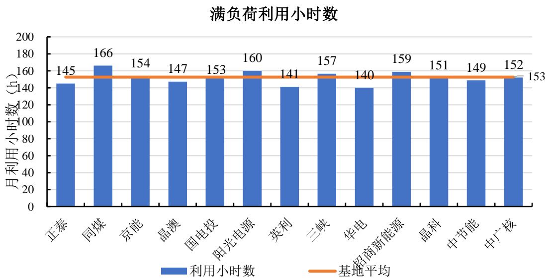
图 6 大同基地各项目满负荷利用小时数
