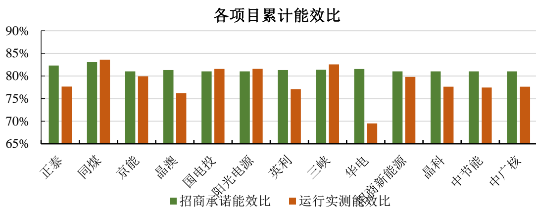
图 13 大同基地各项目当年累计能效比对比图
