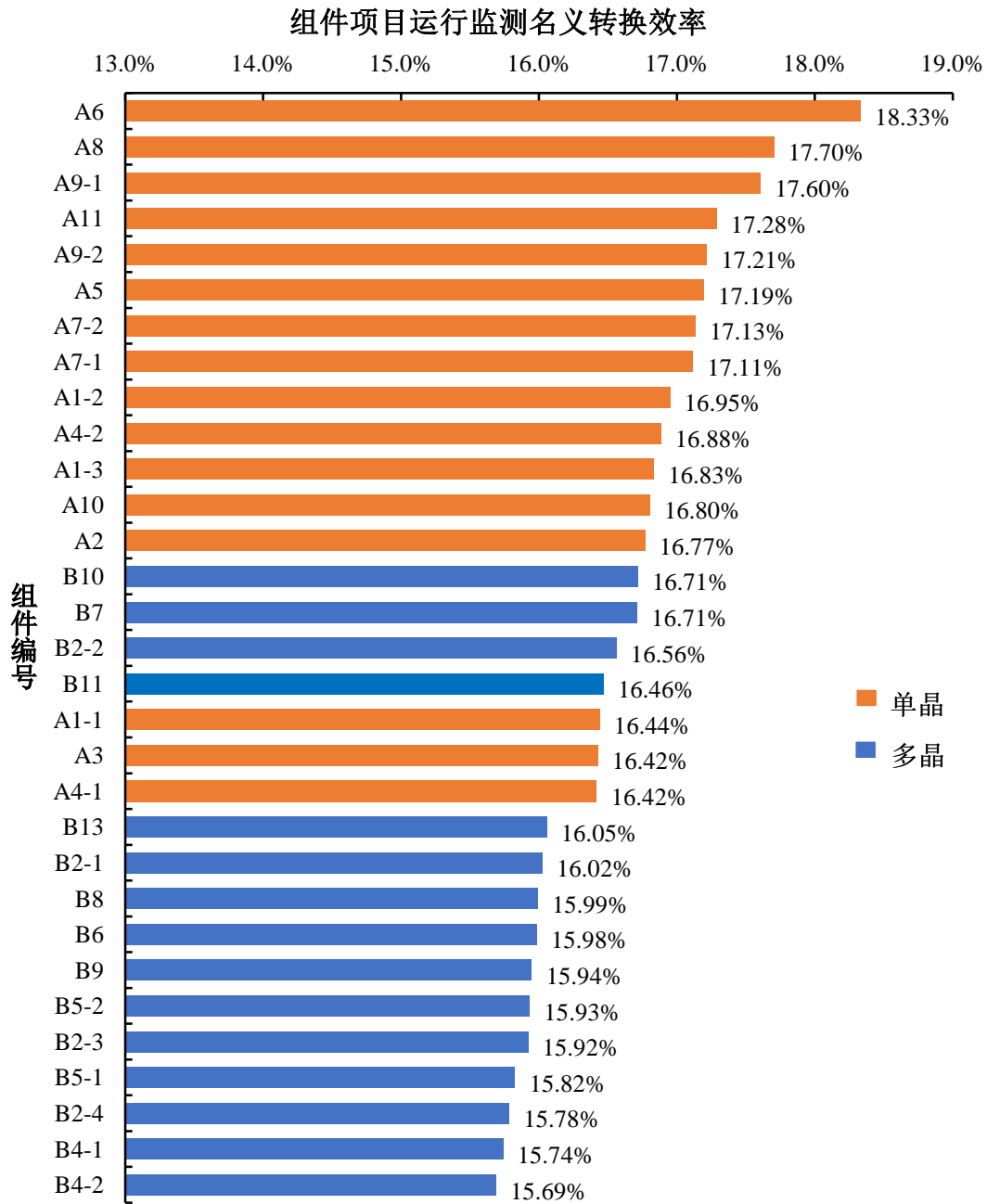
图 8 大同基地组件项目运行监测名义转换效率
