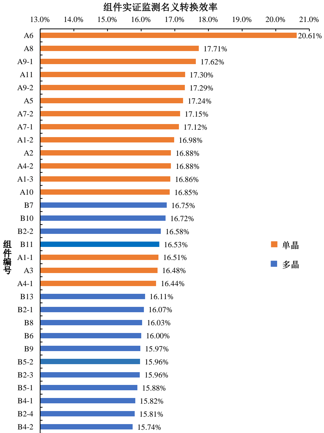
图9 大同基地组件实证监测名义转换效率
