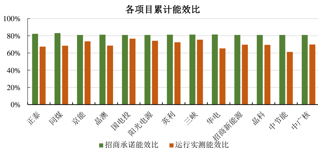
图 13 大同基地各项目当年累计能效比对比
