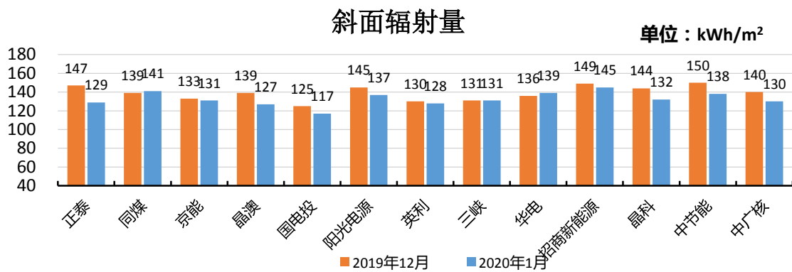
图 1 大同基地各项目斜面辐射量与环比变化
