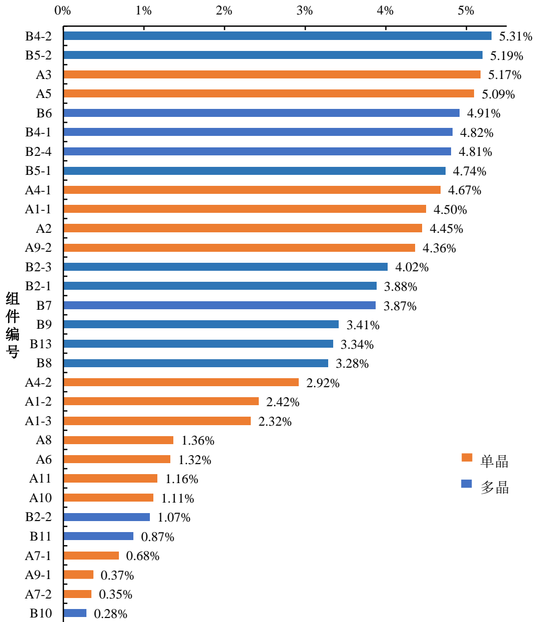
组件项目运行监测功率名义衰减率
