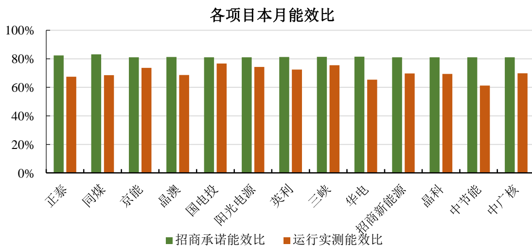
图 12 大同基地各项目本月能效比对比
